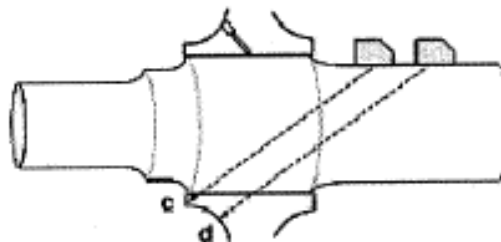
Slika 3. Echo iz područja glavčine točka i prelaznog radijusa glavčine točka.
