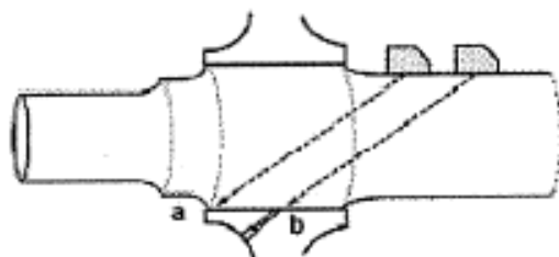
Slika 2. Echo iz područja ivice sjedišta točka i uljnog žlijeba točka.
