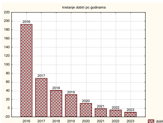
Grafik 1. Kretanje visine dobiti po godinama (polazni podaci).
