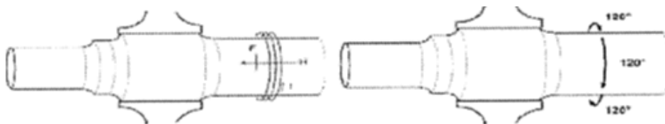
Slika 7. Smjer stvaranja indikacije pomoću strujnog fluksa. Figure 7. Direction of generation of indication using current flux.
