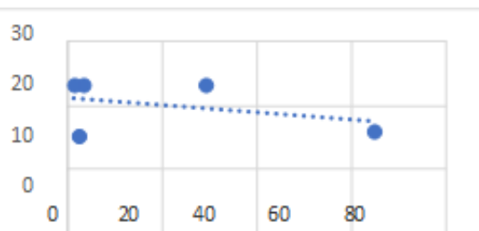
Grafikon 5. Koeficijent korelacije između: Podrška Agencije za razvoj Republike Srpske i Stručna i konsultantska podrška.
